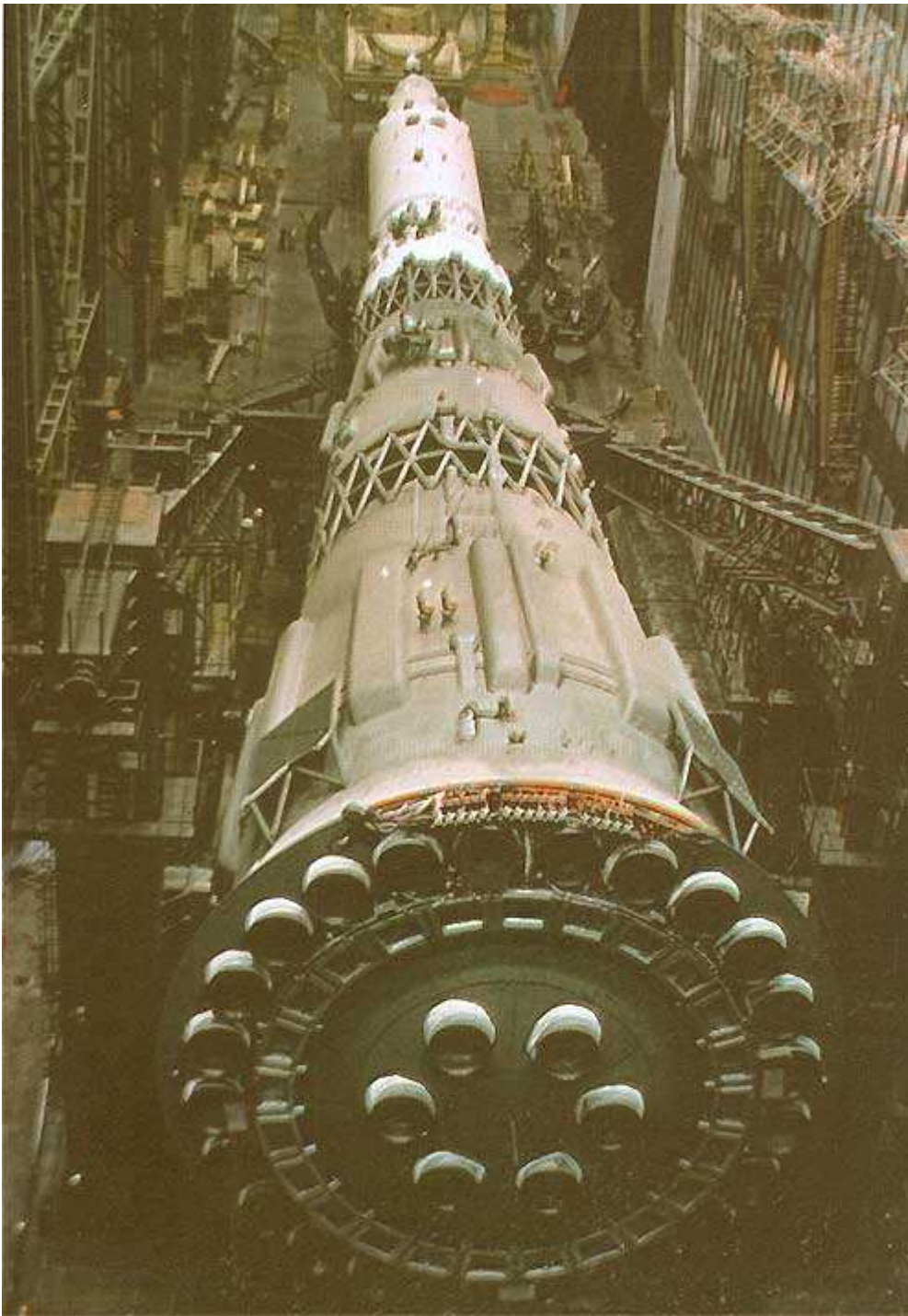
Ракета-носитель Н1 в монтажно-испытательном корпусе. Байконур
