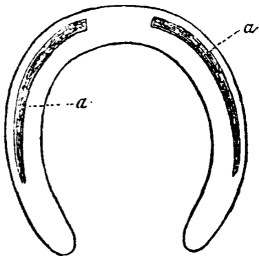
Лѣтняя подкова безъ шиповъ для верховой лошади съ высокими пятками.
