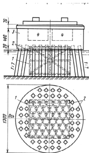
Центральная опора главного разводного пролета Керченского моста
