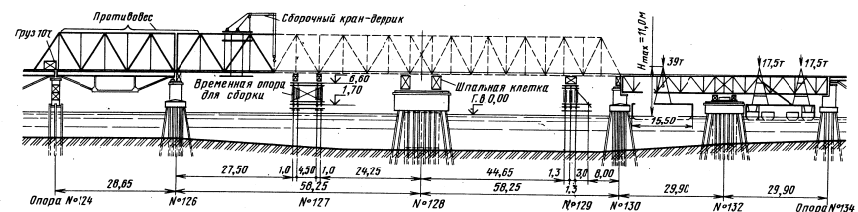
Монтаж разводных пролетов Керченского моста
