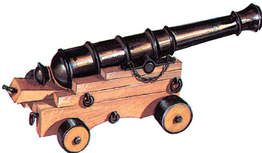
Морская пушка. Морские пушки имели бронзовый (позднее стальной) ствол, поддерживаемый двумя цапфами на деревянном лафете с четырьмя деревянными катками. Когда пушка готовилась к выстрелу, лафет подкатывали к борту судна, чтобы ствол высунулся из пушечного порта. Когда пушку, заряжающуюся с дула, надо было перезарядить, ее откатывали назад, чтобы заложить пороховой заряд, а ядро вкатывалось через дульное отверстие
