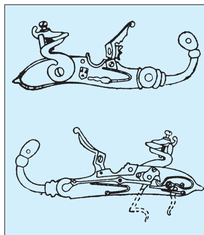
Фитильно-кремневый ружейный замок: наружная (вверху) и внутренняя стороны
