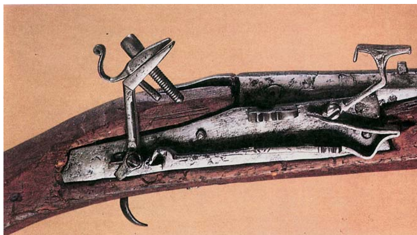
Кремневый замок строевого ружья. Начало XVII в.
