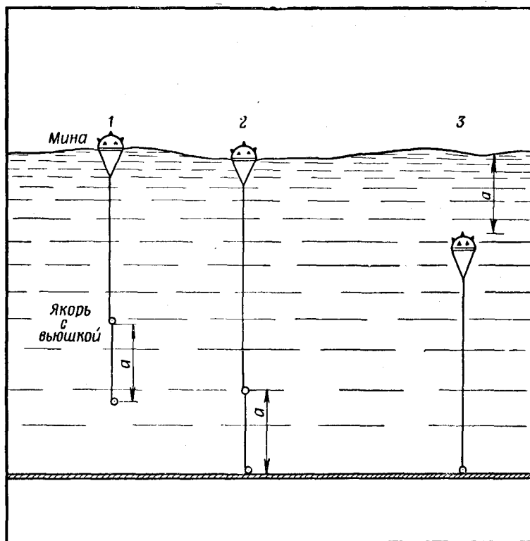
Постановка мин с автоматическим якорем Азарова
