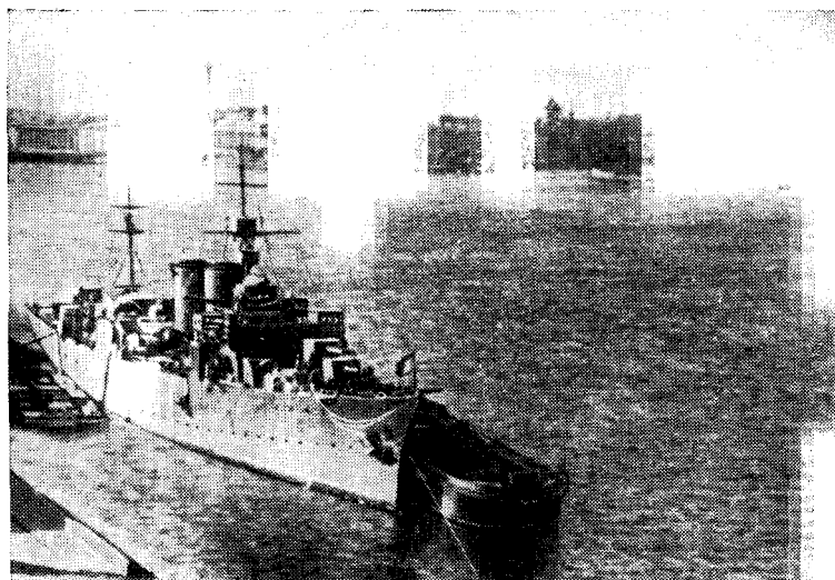
Минный заградитель «Ока»
